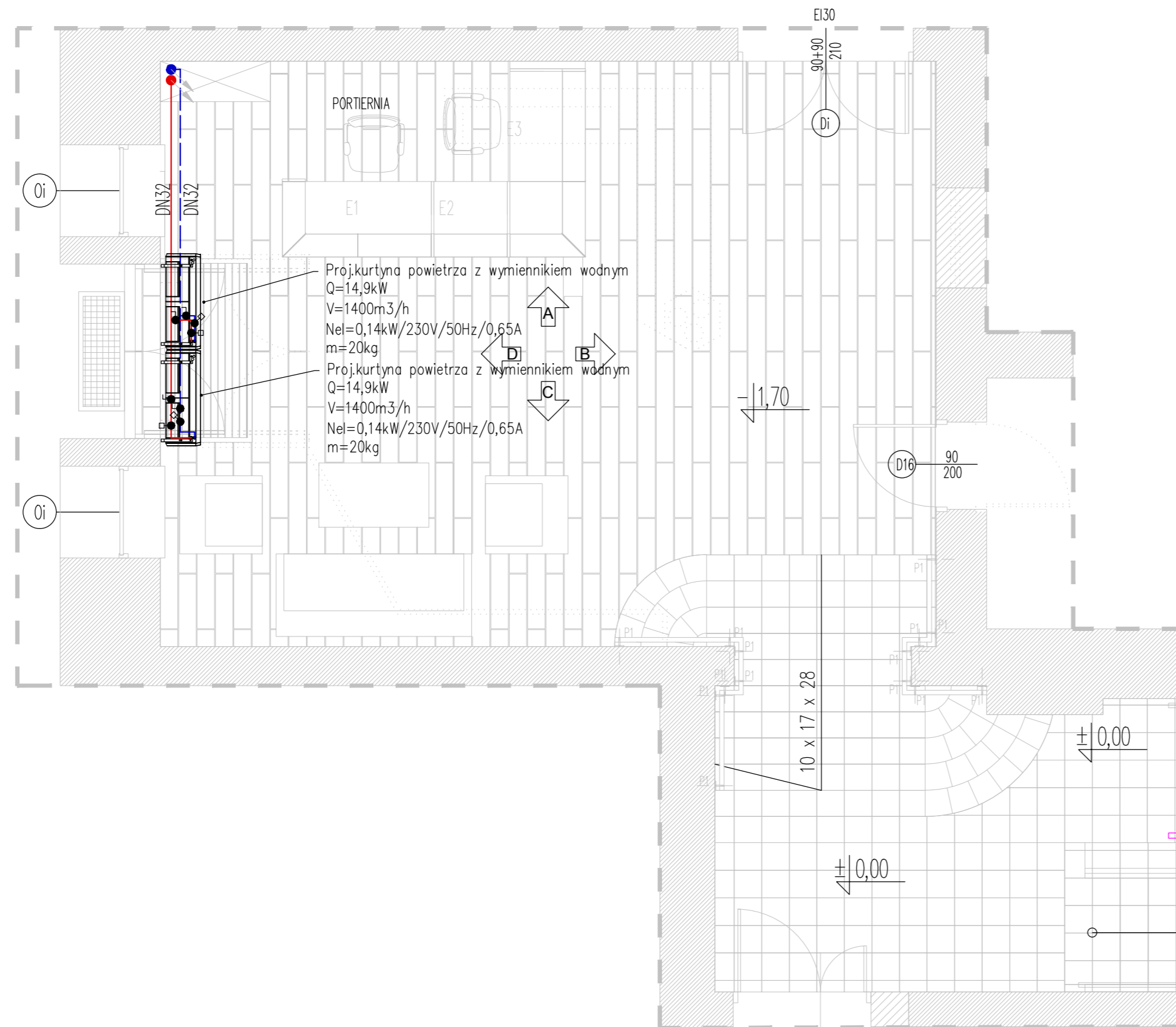
RZUT, SKALA 1:100
