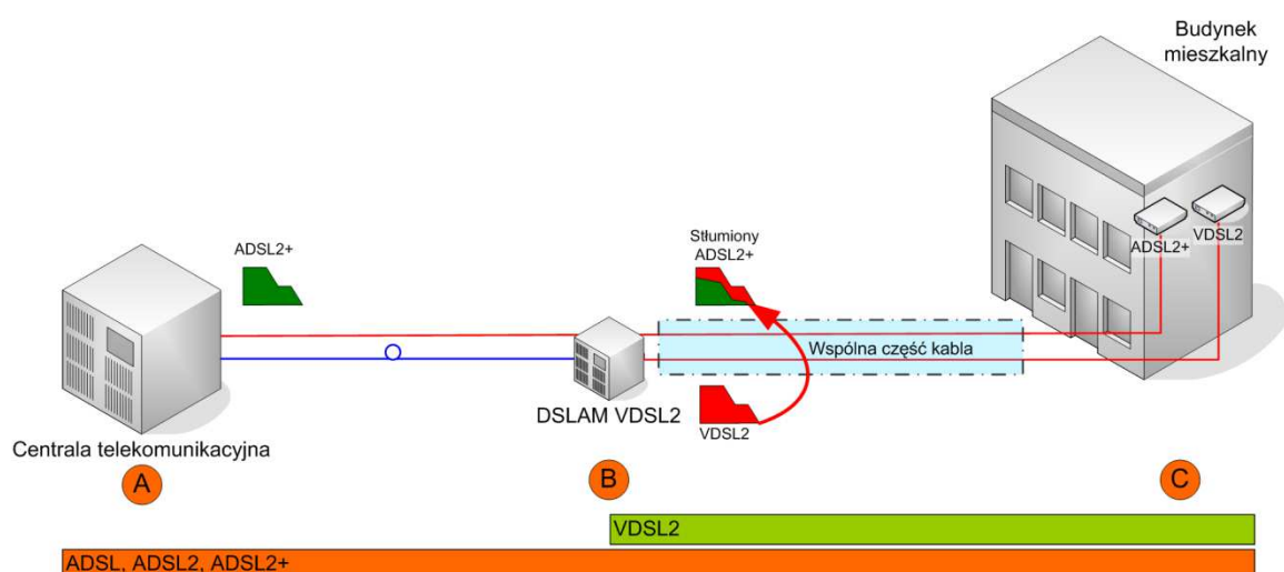
Rysunek 1 Kształtowanie widma w module wyniesionym (na rysunku oznaczonym jako DSLAM VDSL2) jest niezbędne, aby silny sygnał systemu wyniesionego nie wpłynął
