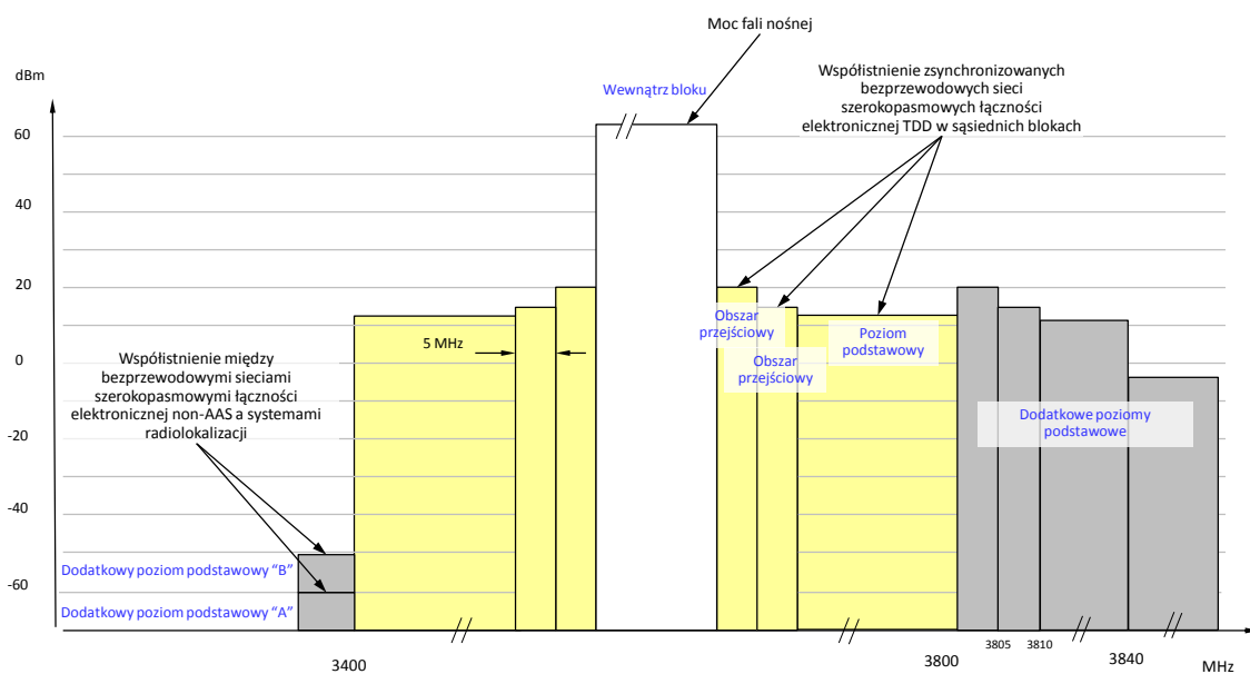
Rysunek 1. Maska BEM dla stacji bazowej obowiązująca dla Ustalonej struktury ramki
